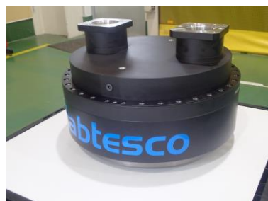
「動くガンダム」用精密減速機RV™
